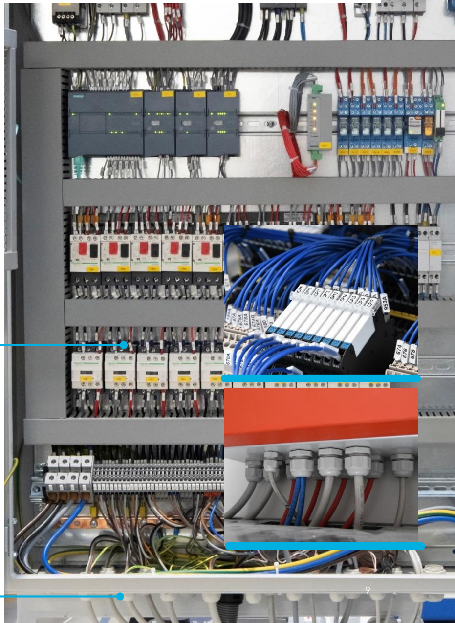
Pressacavi
